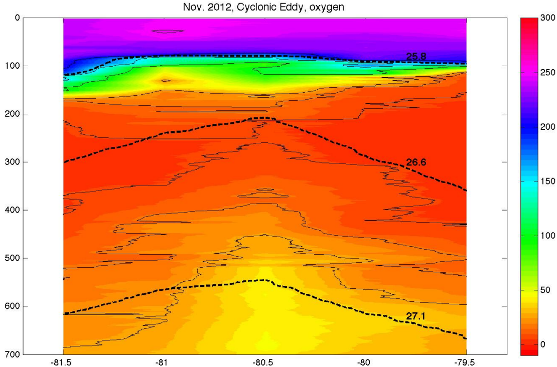
Abb. 1: Sauerstoffverteilung (in \mu mol/kg ) mit einigen ausgewählten Dichtelinien im zyklonalen Wirbel bei ca. 81^\circ W .
