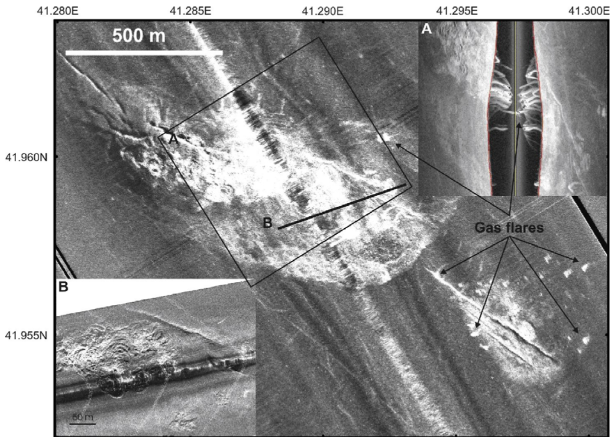
Abb. 7 Mosaik der Sidescan Sonar-Vermessung mit DTS-1 (75 kHz) im Batumi Seep -Gebiet. Hohe Backscatterintensität wird durch hellen Grauton angezeigt. A: Unprozessierte Sidescan-Sonar-Daten zeigen akustische Anomalien in der Wassersäule (Gasblasenaustritte). B: 410 kHz-Aufzeichnung im zentralen Seepbereich. (aus Klaucke et al. 2006, Marine Geology 231, 51-67)
