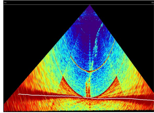
Abbildung 5: Abbild der Gasaustritte durch die Wassersäule, aufgezeichnet mit dem EM710 Fächerlot an der gleichen Position wie im Bild 4 zu sehen.
