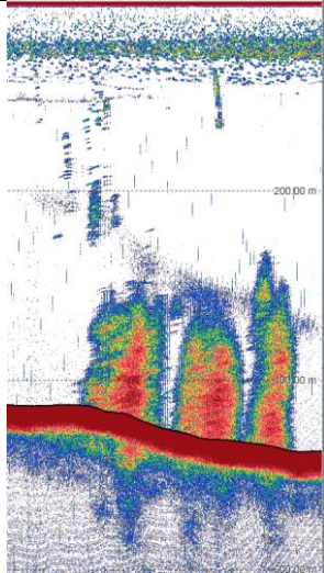
Abbildung 4: Beispiel von einem akustischen Abbild von Gasaustritten, welche mit dem EK80 System aufgezeichnet wurden.
