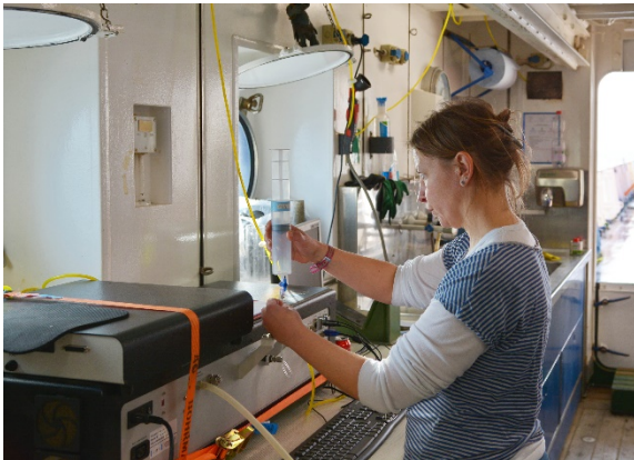
Abbildung 1: im Geolabor der METEOR misst Dr. Susan Mau mit dem Laser-basierten ICOS-Meßgerät die Treibhausgase CO 2 und CH 4 in Luft und Wasser (© A. Popa).
