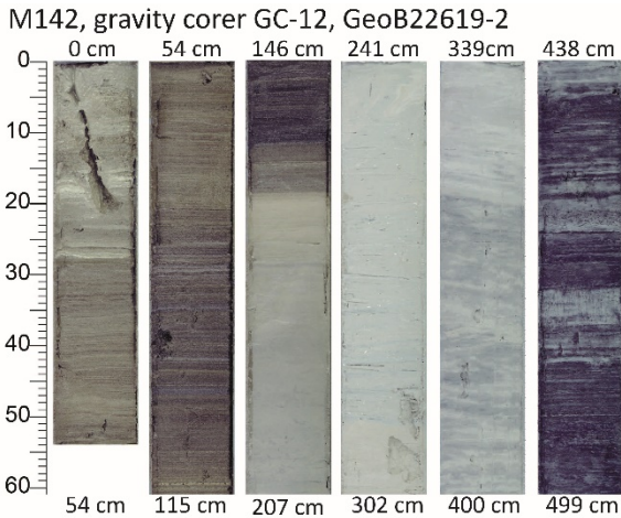
Abbildung 3: Jüngste Sedimentabfolge des Schwarzen Meeres. Unter Coccolithenschlämmen (0-27 cm) folgt ein laminierter Sapropel (28-165 cm), der von Seesedimenten mit dunklen bis schwarzen Eisensulfid-Verfärbungen unterlagert wird.
