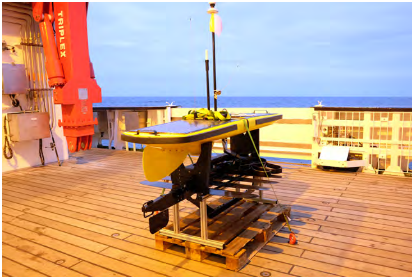
Wellenleiter GeoSURF fertig zum Einsatz an Deck des FS SONNE.
