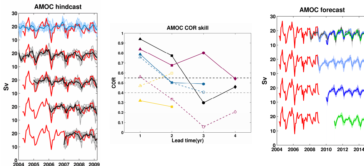
Abb. 4.2.1: (Links) AMOC-Stärke: zonal integrierter nordwärtiger Transport bei 26.5^\circ N oberhalb von 1000m. Die beobachteten Transporte stammen von RAPID/MOCHA (rot), die individuellen "Nachhersagen" und ihr Ensemblemittel sind in Grau und Schwarz dargestellt. Transporte der nicht-initialisierten Simulation sind in hell- bzw. Dunkelblau dargestellt. (Mitte) Vorhersagegüte dargestellt als Korrelationskoeffizient (COR) für Startdatum Jan 2004 (schwarz), Jan 2005 (violett), Jan 2006 (blau) und Jan 2007 (orange) als durchgezogene Linien. Die entsprechenden Werte für die Persistenzvorhersage erscheinen als gestrichelte Linien. (Rechts) RAPID/MOCHA Zeitreihen (rot) und die AMOC Vorhersagen für die Startdaten Jan 2008 (grau/schwarz), Jan 2009 (hellblau), Jan 2010 (dunkelblau) und Jan 2011 (grün).
