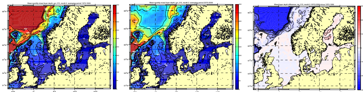
Abb.8: Änderungen der Deckschichttiefe links: 1970 – 1999; Mitte: 2070 – 2099; rechts: Differenz
