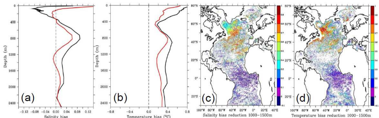
Abb. 4: Salzgehalts- (a) und potentieller Temperaturbias (b) von der Simulation (schwarz) und dem optimierten Modell (rot). (c, d) Reduktion des Salzgehalts- und des potentiellen Temperaturbias in der Schicht 1000-1500m.
