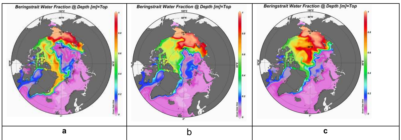
Abbildung 10: Konzentration eines künstlichen Tracers für Pazifikwasser (Bering Strait Water) an der Oberfläche in den Jahren (a) 1997, (b) 2000 und (c) 2004.
