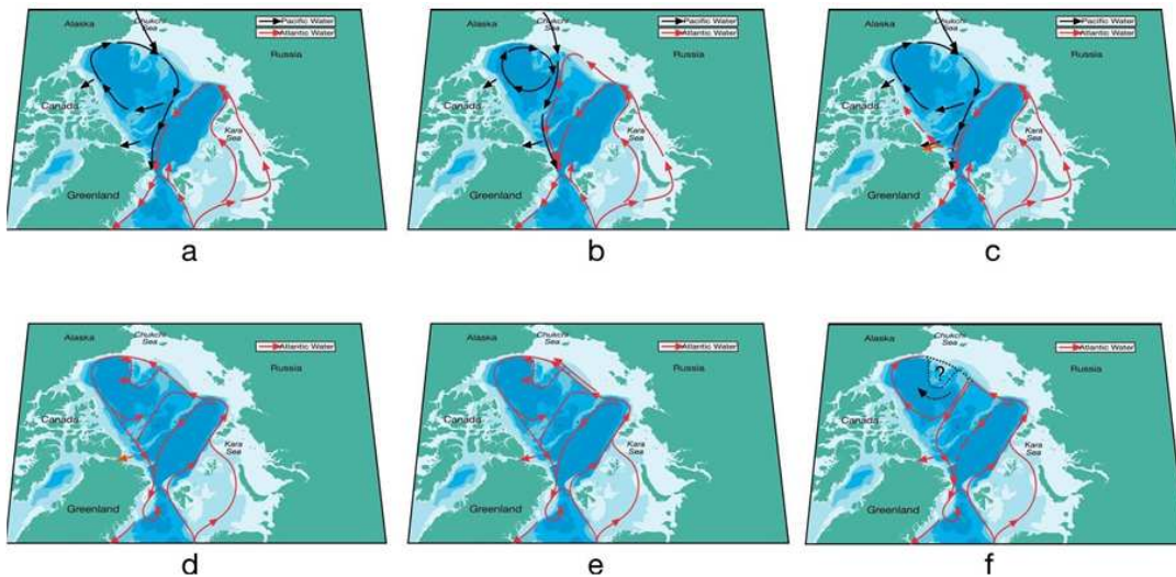
Abbildung 9: Zirkulationsschema für Wasser atlantischen (rot) sowie pazifischen Ursprungs (schwarz). Oberflächenströmungen in den (a) 1980er Jahren, (b) in den 1990er Jahren, (c) nach 2004 (gestrichelte Linien zeigen intermittierende Strömungen; Strömungen der Atlantischen Wasserschicht in den (d) 1980er Jahren, (e) 1990er Jahren (doppelte Pfeile im Makarow- und Kanadabecken zeigen verstärkten Transport im Randstrom), (f) nach 2004. Die gestrichelte Linie entlang des Lomonosov Rückens zeigt abgeschwächte Strömung Atlantischen Wassers. Unklare Strömungsverhältnisse: gepunktet und mit Fragezeichen versehen. Schwarzer gepunkteter Pfeil: Einstrom Atlantischen Wassers mit hohen Jodkonzentrationen in das zentrale Kanada-becken. Nach 2004 Wechsel zu einem sehr starken antizyklonalen Regime an der Oberfläche mit Umkehr der Zirkulation der Atlantischen Wasserschicht im Kanadabecken.
