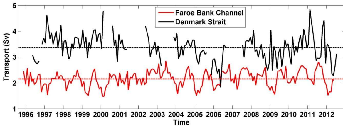
Abb. 1: Zeitreihen der aus den Daten von verankerten Strömungsprofilmessern bestimmten Volumentransporte des Färöer-Bank-Kanal-Overflows (rot) und des Dänemarkstraßen-Overflows (schwarz).
