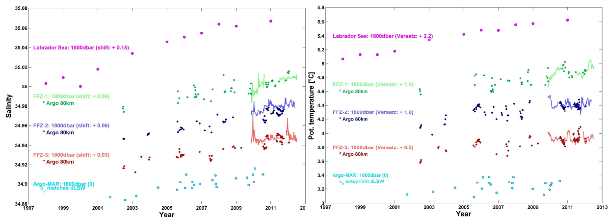
Abb. 2: Zeitreihen des LSW-Salzgehalts (1800 dbar) aus den FBZ-Verankerungen am Mittelatlantischen Rücken (Linien) und aus Argo-Profilen (Punkte), die maximal 80 km entfernt von der Verankerungsposition gemessen wurden. Des Weiteren die Jahresmittelwerte aus der Labrador See (Magenta) und Argo-Messungen direkt über dem MAR (Cyan). Zur besseren Sichtbarkeit wurden die Zeitreihen vertikal versetzt abgebildet.
