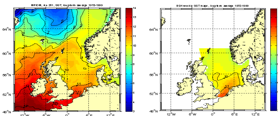
Abb. 3: Klimatologisches Mittel der Oberflächentemperatur für den Zeitraum 1970 – 1999. Links: ungekoppelter Hindcastlauf, rechts: Mittel aus den wöchentlichen Oberflächentemperaturanalyse des BSH
