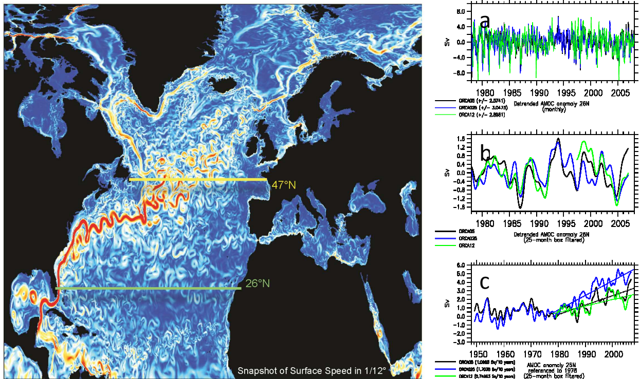
Abb. 8: Links: Momentaufnahme des Betrags der Oberflächengeschwindigkeit im globalen 1/12^\circ Modell (ORCA12). Rechts: Schwankungen der meridionalen Umwälzbewegung (MOC) in 26^\circ\text{N} (in Sv) in den Hindcast-Simulationen mit den 1/2^\circ , 1/4^\circ und 1/12^\circ Modellversionen, (a) Zeitserien von Monatsmittelwerten, (b) tiefpass-gefiltert, relativ zum linearen Trend des jeweiligen Modells; (c) Monatsmittelwerte, relativ zum MOC-Transport im Jahr 1978.
