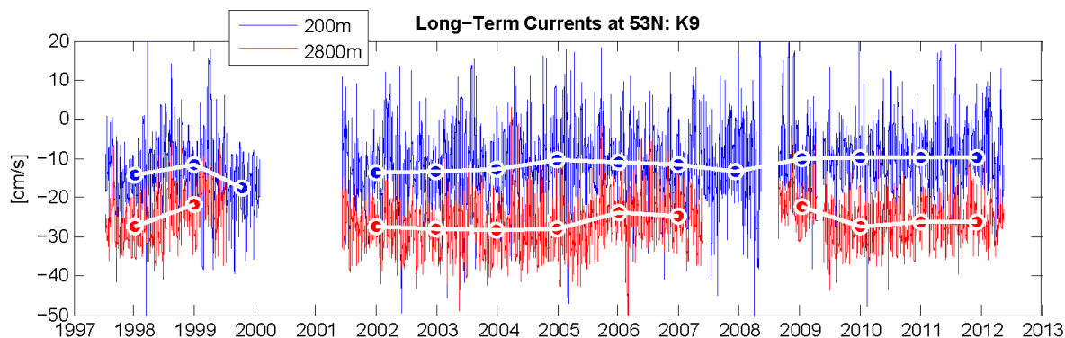
Abb. 6: Zeitserien (hochaufgelöst und Jahresmittel) der Strömungen an der zentralen Station (K9) des 53°N-Observatoriums. In Blau die oberflächennahen S Strömungen und in Rot die wesentlich stärkeren Strömungen im tiefen DSW-Kern des Randstroms.
