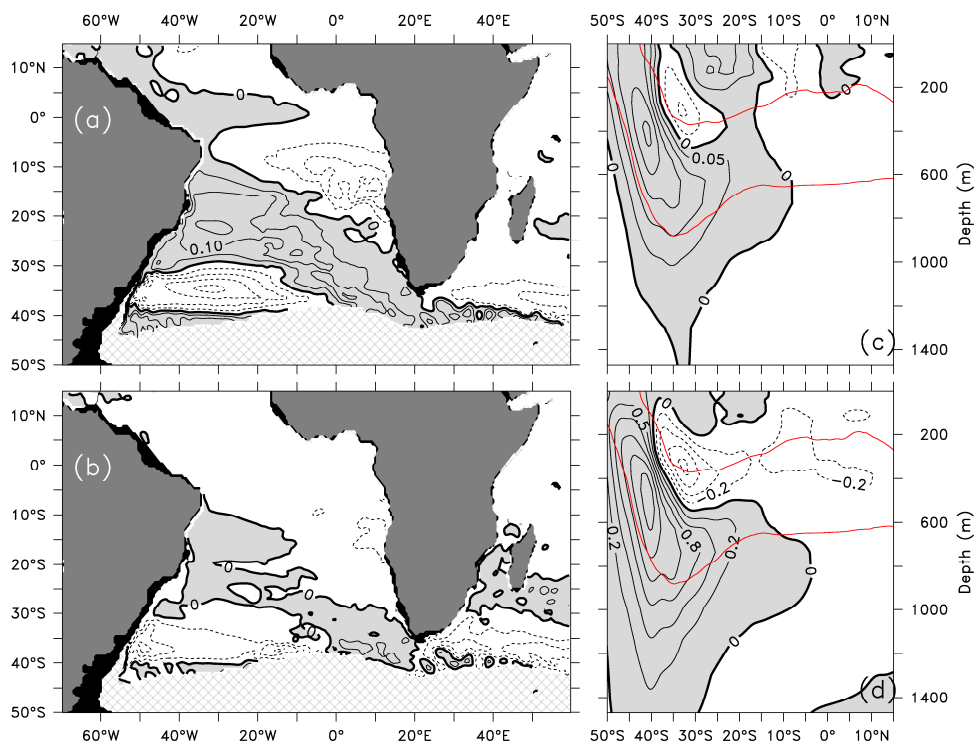
Abb. 10: Wassermassenänderungen im Atlantik durch Änderungen der südhemisphärischen Windsysteme. (a) Salzgehalts- und (b) Temperaturänderungen in der oberen Thermokline. Änderungen im zonalen Mittel von (c) Salzgehalt und (d) Temperatur im Atlantik. (Abb. aus Biaستoch und Böning, 2013).
