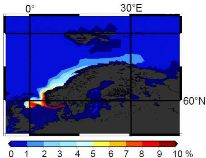
Abb. 4: Anomalie an gelöstem anorganischen Kohlenstoff in rd. 100m Wassertiefen in einer Modellsimulation in der die atmosphärische \text{CO}_2 Konzentration ausschließlich über der Nordsee auf den 4-fachen vorindustriellen Wert festgeschrieben wurde. Dargestellt ist das Mittel über die letzten 5 Jahre einer Modellintegration über 20 Jahre.
