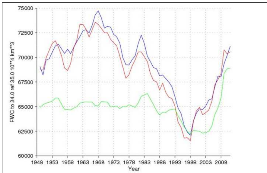
Abbildung 6: Süßwassergehalt des Nordpolarmeeres im NAOSIM Hindcast-Experiment 1948-2010: gesamter Bereich (blau), Bereich mit Wassertiefen > 500 m (rot) und im Beaufortwirbel (grün). Letztere sind mit einem Versatz von +23000 \text{km}^3 bzw. +50000 \text{km}^3 versehen um eine gemeinsame Darstellung zu ermöglichen.
