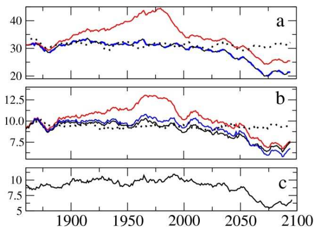
Abb.3: Jährliche Primärproduktion und b) Netto-Kohlenstoffaufnahme in der Nordsee (Mio. Tonnen Kohlenstoff.) Gestrichelt=Kontrolllauf ohne Klimaerwärmung, Schwarz=mit Klimaerwärmung, blau= wie schwarz + CO 2 Anstieg in der Atmosphäre, rot= wie blau + anthropogene Nährstoffeinträge über Flüsse. c) Nährstofftransport (gelöstes Nitrat in kmol/s) vom Nordatlantik über die Schelfkante in die Nordsee.
